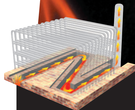
Principe de chauffe
